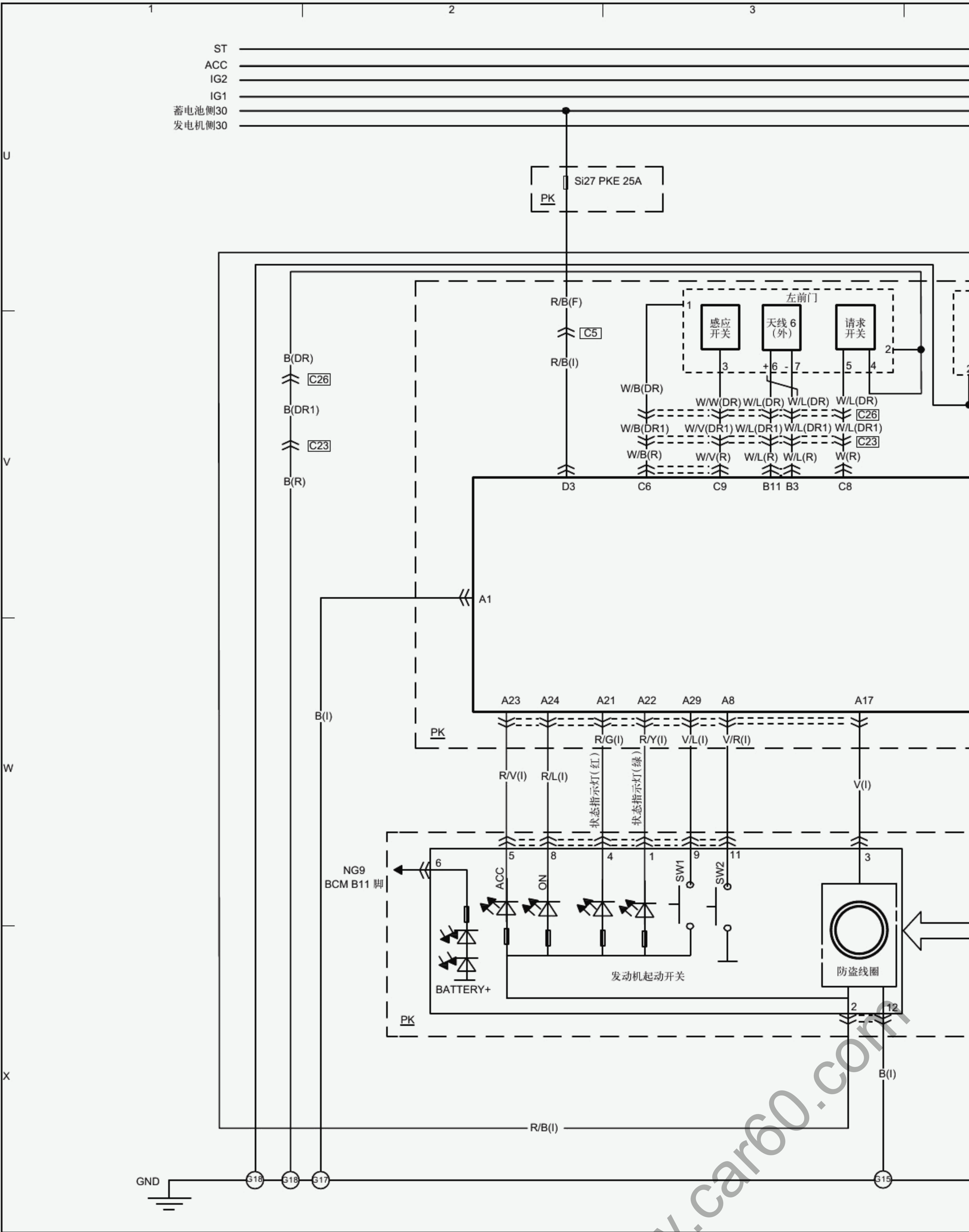
M 总电路图-6
